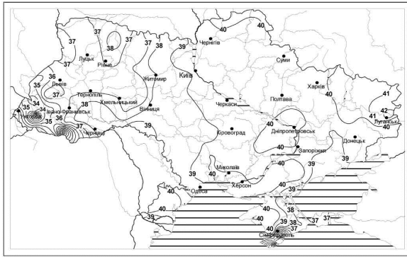
Рис. 1. Абсолютний максимум температури повітря (°C) за 2005–2017 рр.
